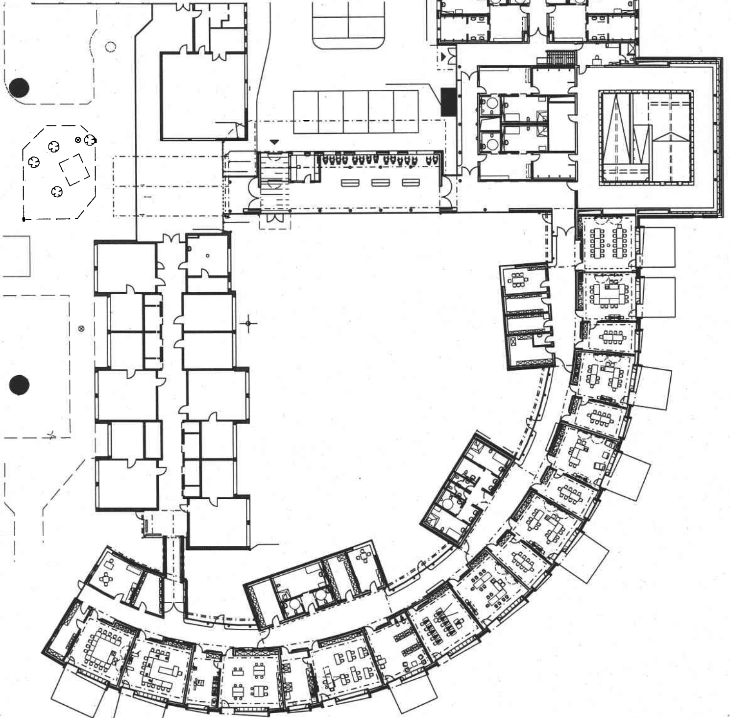
Erdbgeschoss o.M.
