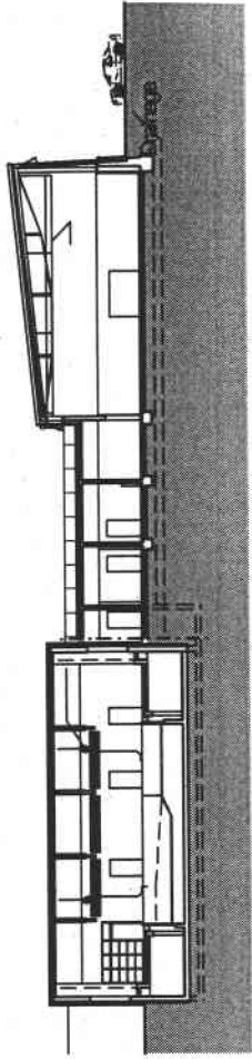
Schnitt Schwimmhalle/ Turnhalle o.M
