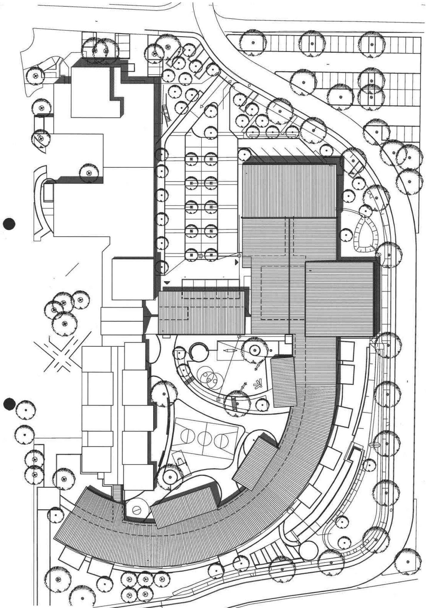
Lageplan o.M
